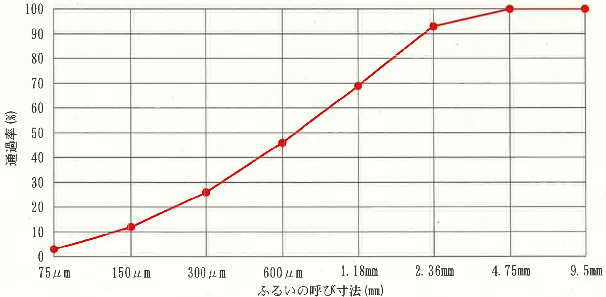
粒度曲線
